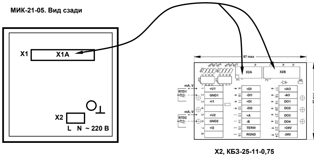
Рисунок Б.1 - Подключение клеммно-блочного соединителя КБ3-25-11-0,75 к регулятору МИК-21-
