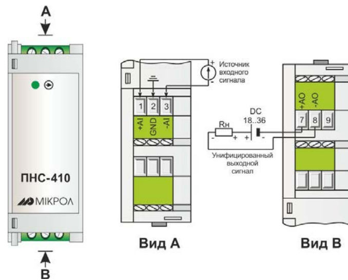
Рисунок 4.3 - Схема электрических подключений
