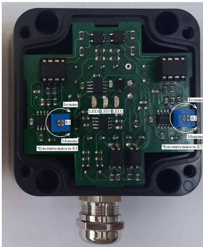
Рис.1 Вид со снятой крышкой.
