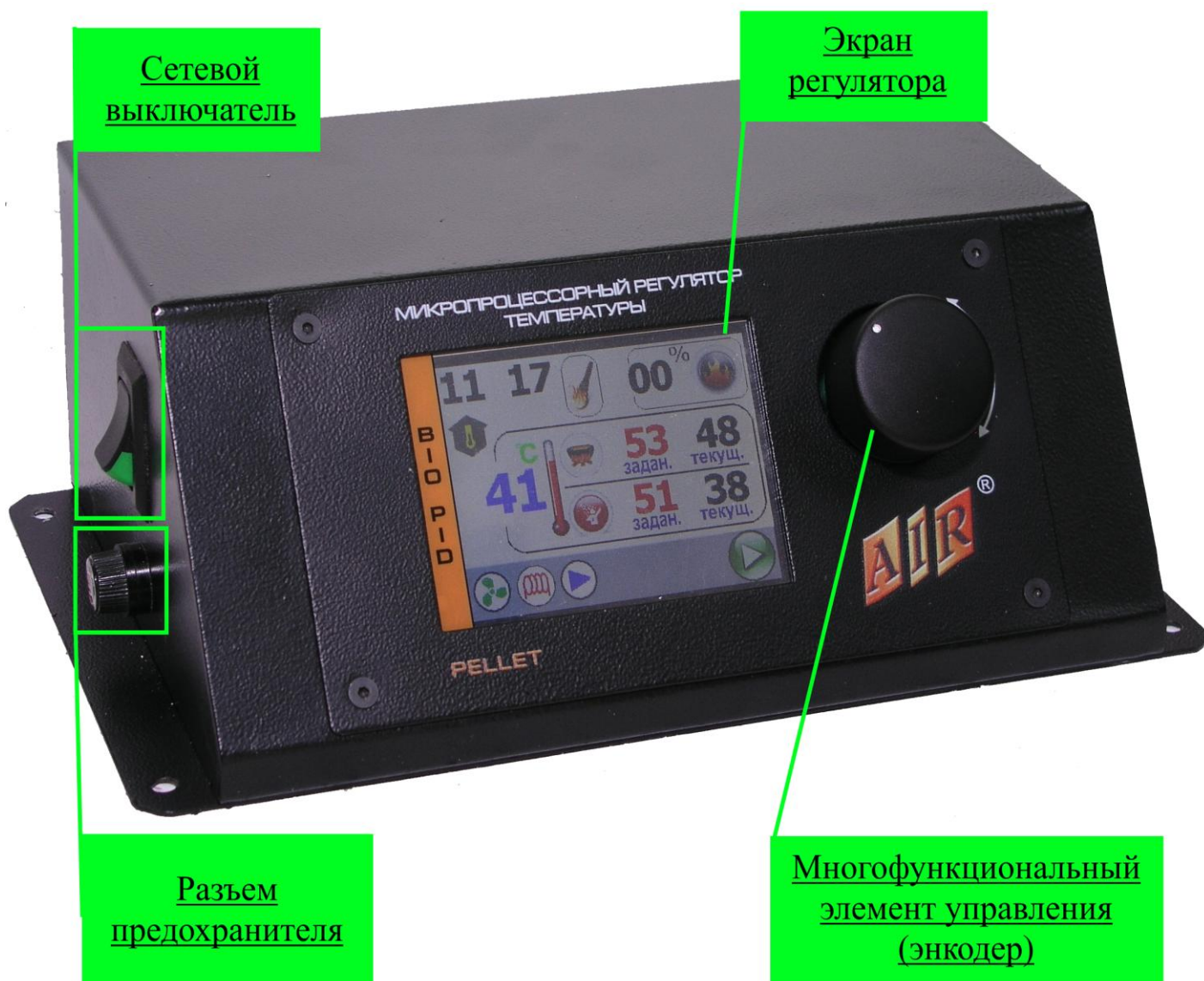
Рисунок 3 – Внешний вид контроллера
