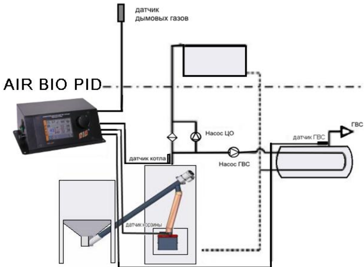
Рисунок 2 – Схематическое расположение датчиков температуры
