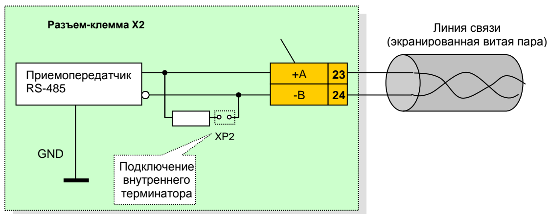
Рисунок Б.5 - Схема подключения внутреннего терминатора
