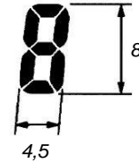
Рисунок А.1 – Внешний вид и размеры цифровых индикаторов регулятора МИК-112
