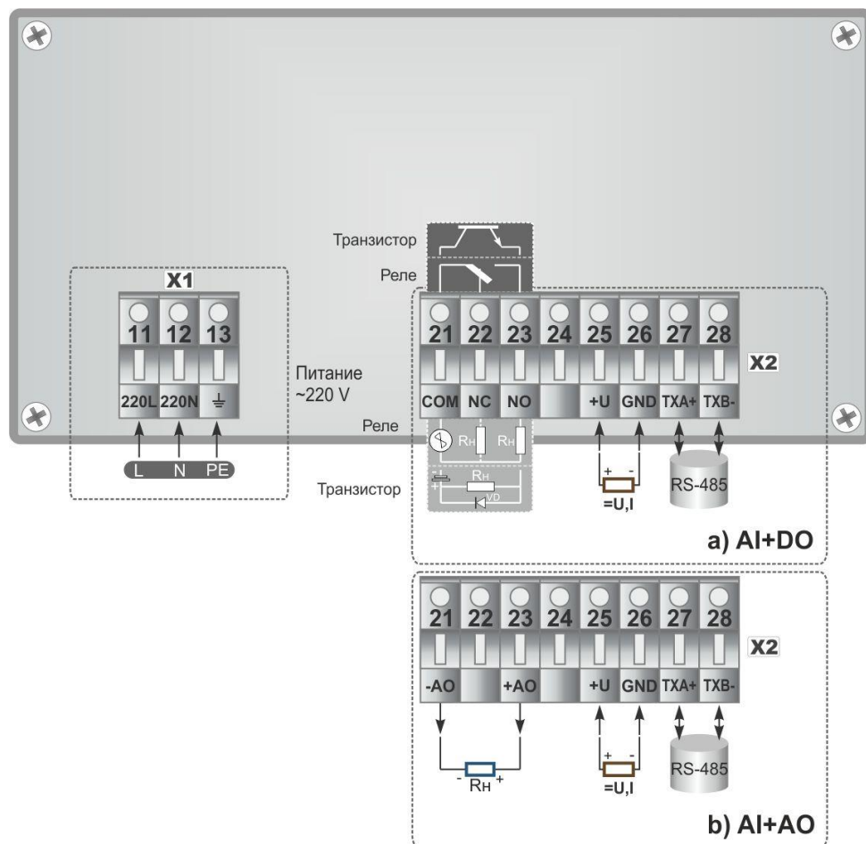
Рисунок Б.1 - Подключение внешних цепей к вольтметру ИПМ-1:
