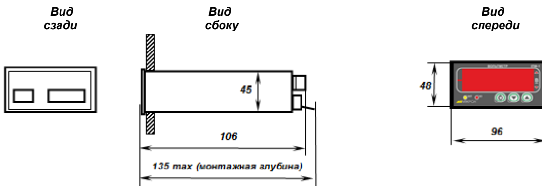
Рисунок А.1 – Внешний вид вольтметра ИПМ-1
