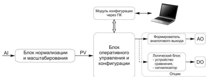
Рисунок 3.3 - Функциональная схема вольтметра ИГМ-1
